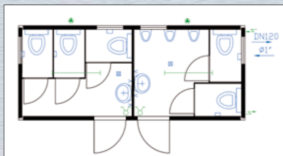
Exemple de plan de base - 20' WC H/F
