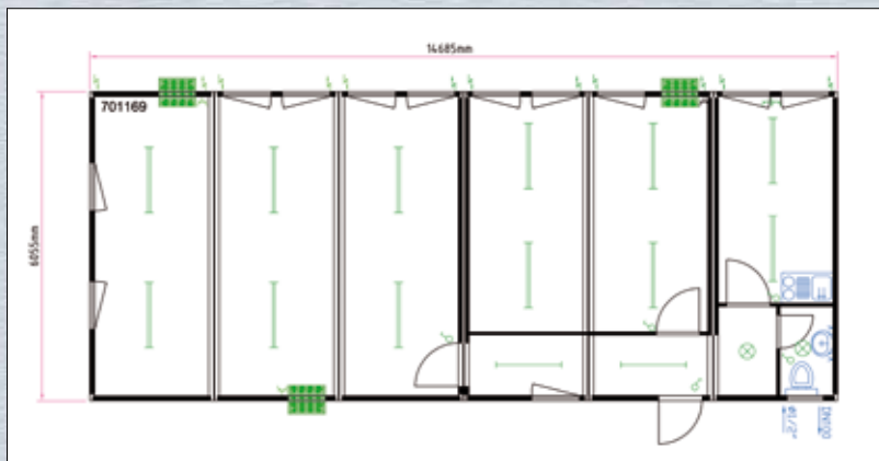
Exemple de plan de base - ensemble de 6
