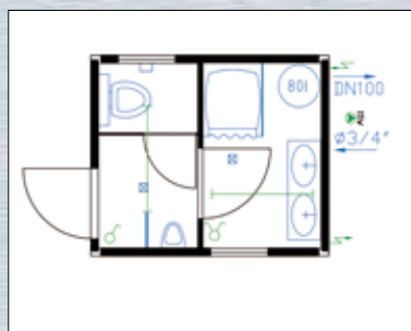
Exemple de plan de base - SA 10'
