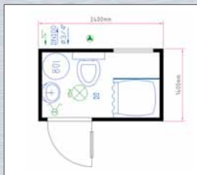
Plan de base - conteneur WC / douche 8'
