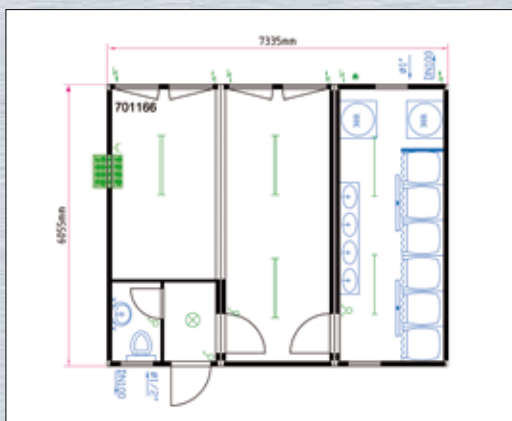
Exemple de plan pour ensemble triple
