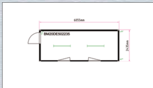
Plan d'un BM 20'standard
